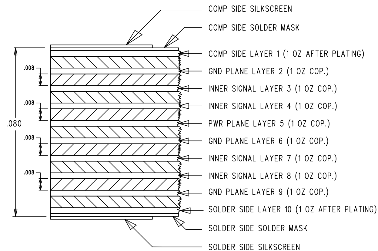
10 LAYER DETAIL
